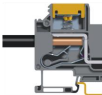
接続完了
