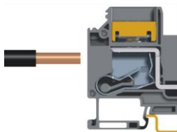
電線挿入
